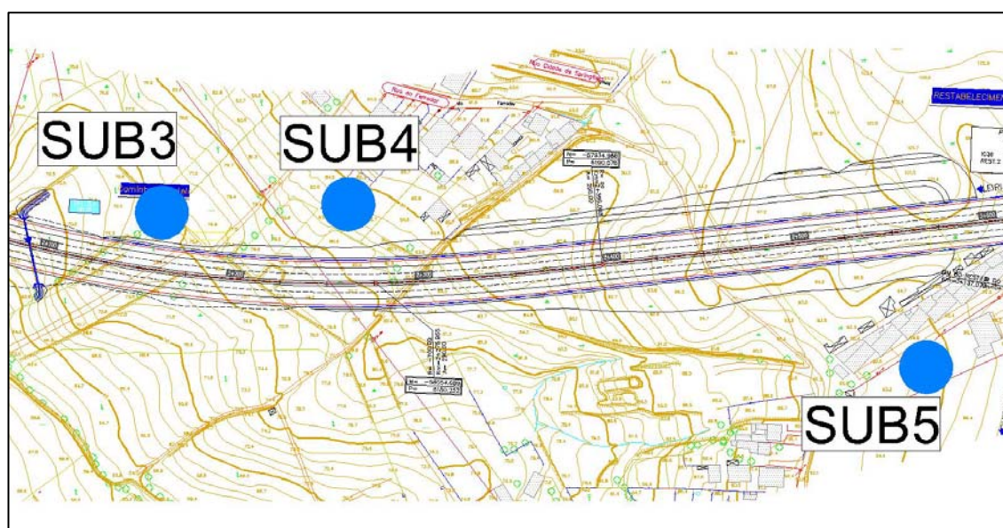
Figura 14 – Pontos de monitorização SUB3, SUB4 e SUB5, localizados aos km 2+175, 2+225 e 2+500, respetivamente
