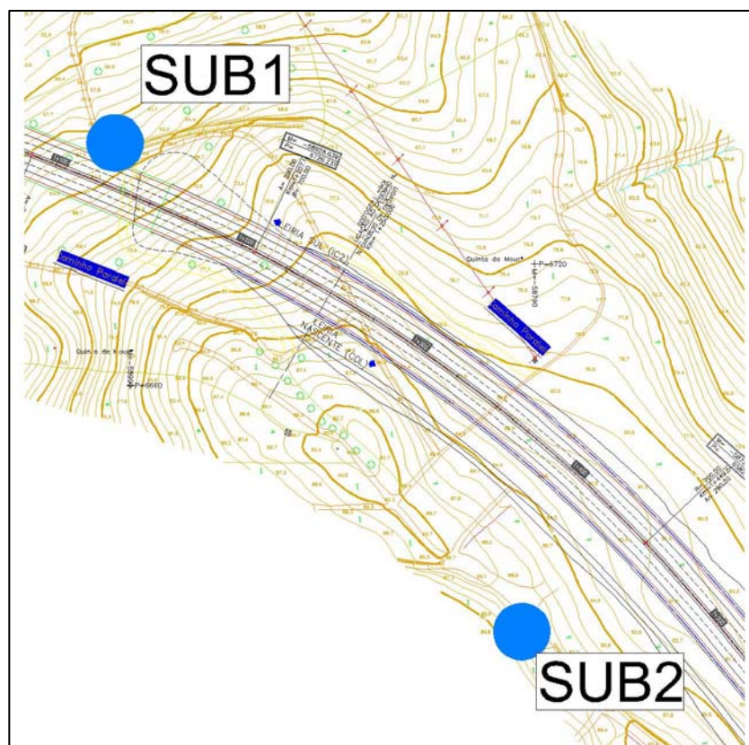
Figura 13 – Pontos de monitorização SUB1 e SUB2, localizados aos km 1+100 e 1+450, respetivamente
