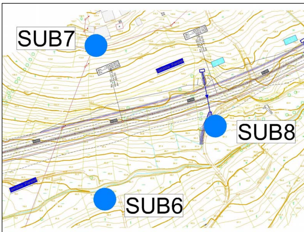
Figura 15 – Pontos de monitorização SUB6, SUB7 e SUB8, localizados aos km 4+950, 4+900 e 5+125, respectivamente
